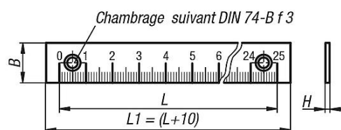
Avec perçages position d'implantation verticale
